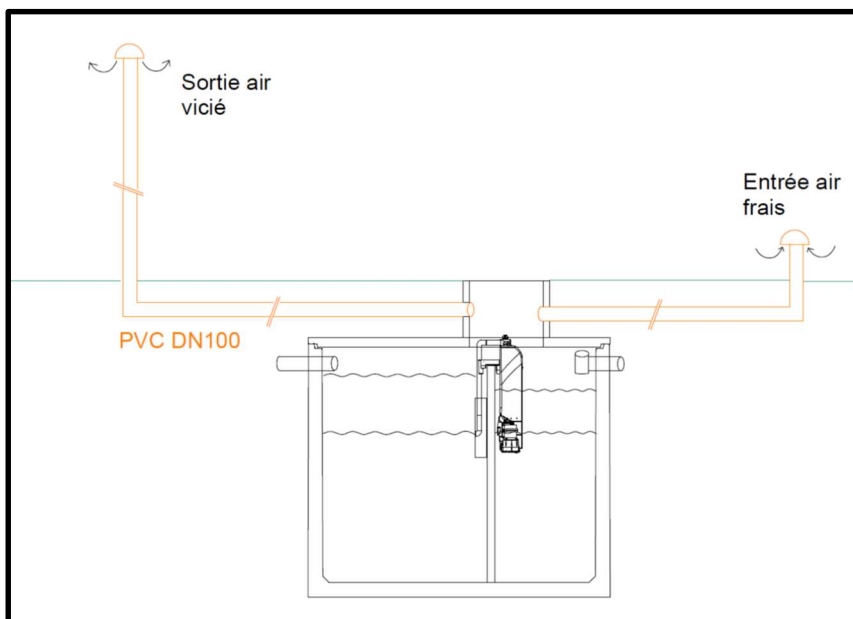
Schéma de principe non contractuel
